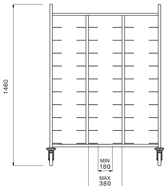
Zij aanzicht
